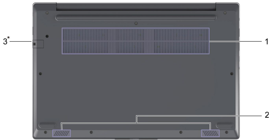
图 8. 底视图—14 英寸型号
