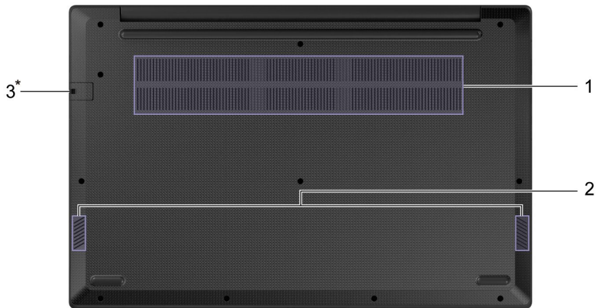
图 9. 底视图—15 英寸型号
